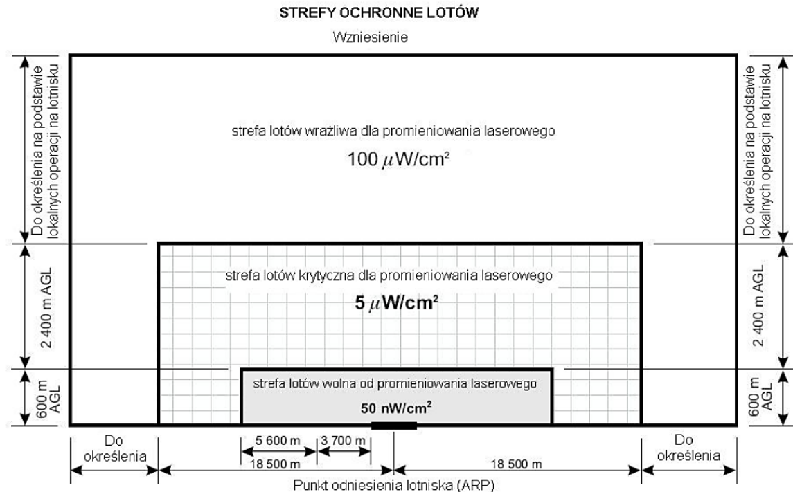
Rysunek 5-13. Strefy ochronne lotów ze wskazaniem maksymalnych poziomów widzialnego promieniowania laserowego
