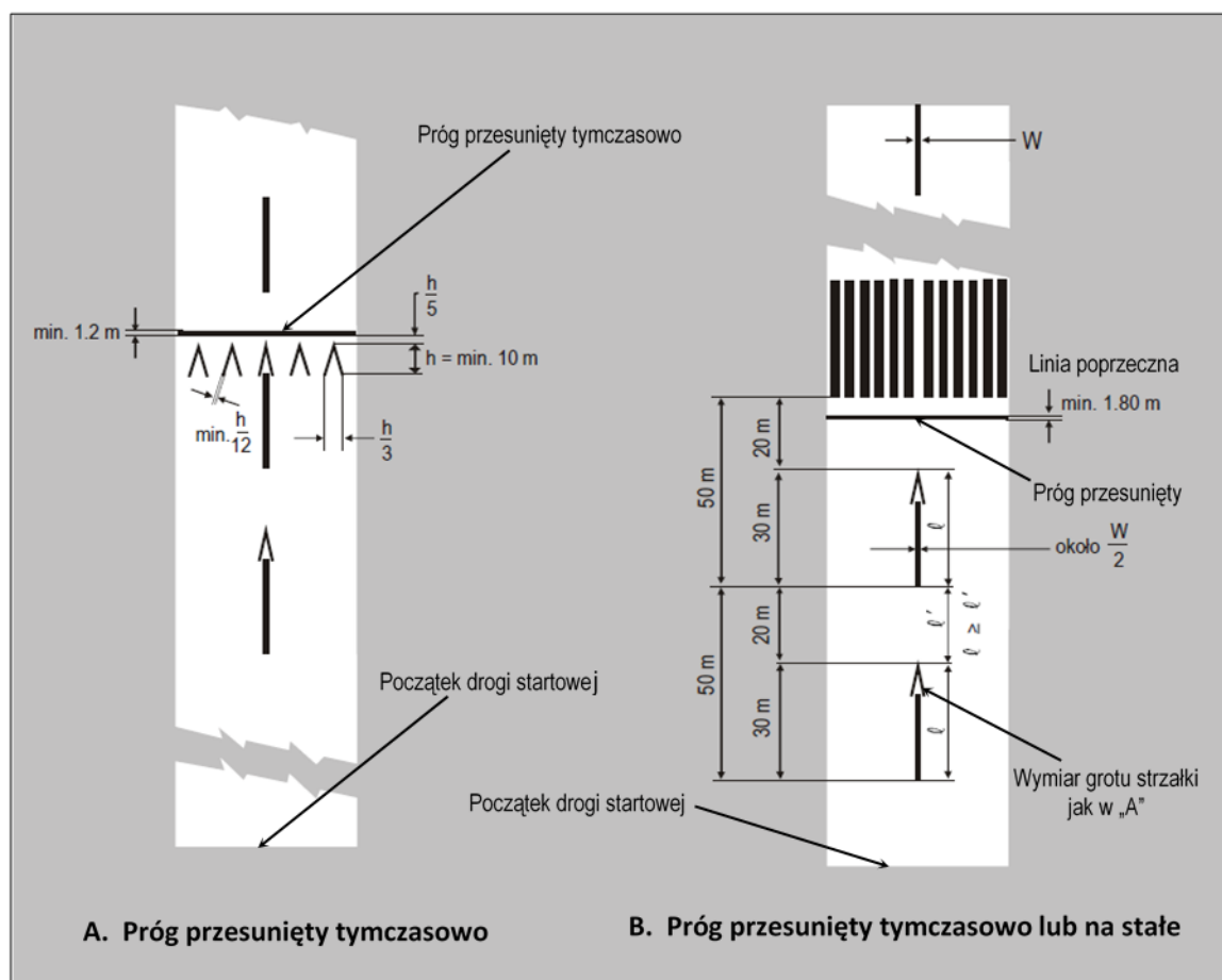
Rysunek 5-4. Oznakowanie przesuniętego progu
