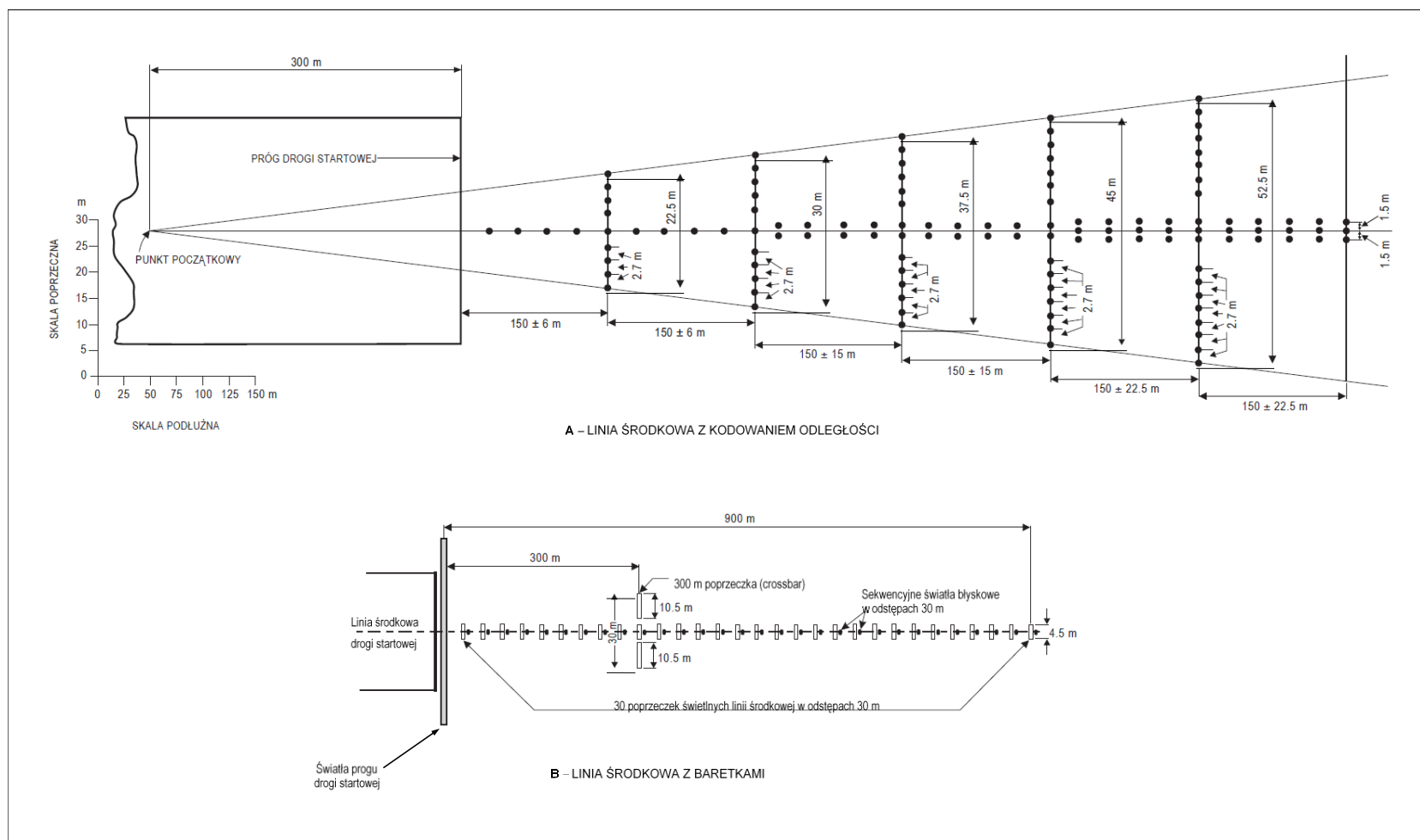
Rysunek A-8. System świateł podejścia precyzyjnego kategorii I
