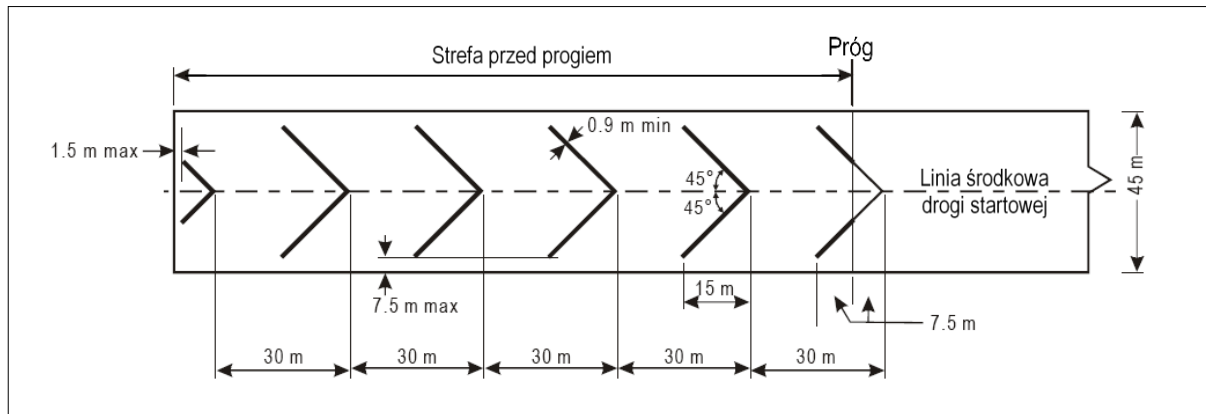
Rysunek 7-2. Oznakowanie powierzchni przed progiem drogi startowej
