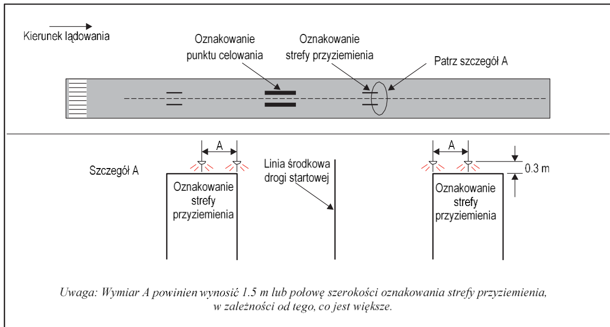
Rysunek 5-24. Proste światła strefy przyziemienia
