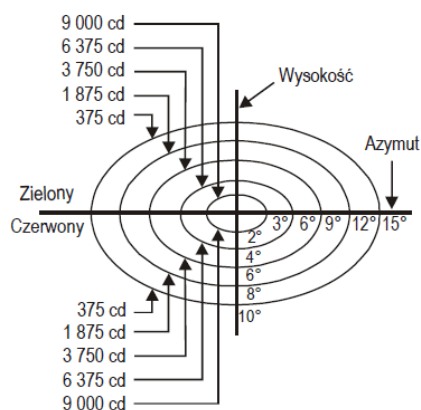
Ilustracja 4 – System HAPI
