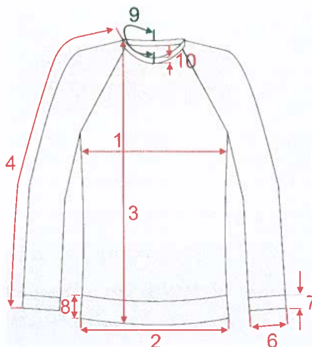
Rys. nr 1. Wymiary wyrobu gotowego zbierane w stanie swobodnym.
